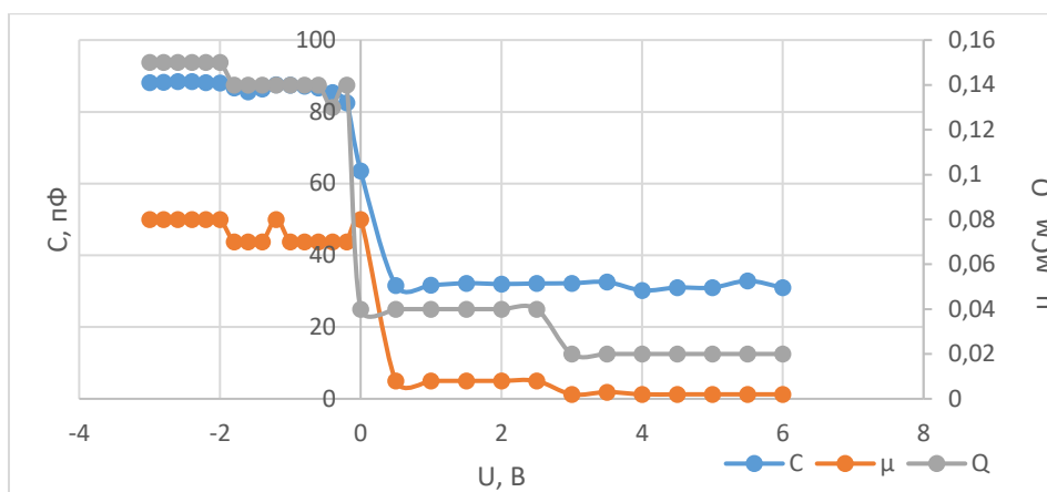
Рис.1. Вольт-ёмкостные характеристики \text{GdF}_3\text{-pSi} , проводимости и тангенса угла диэлектрических потерь от напряжения для толщины диэлектрика d=0,17 мкм
