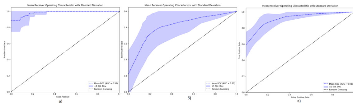
Рисунок 1 – ROC-кривые для идентификации почечной недостаточности методом случайного леса(а), градиентного бустинга(б) и многослойного перцептрона(в)
