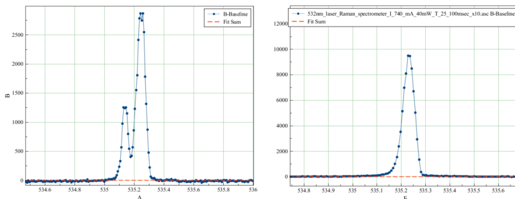
Рис. 1. Спектр лазерного диода с длиной волны 532 нм а) при температуре лазера 20°C б) при температуре 25°C
