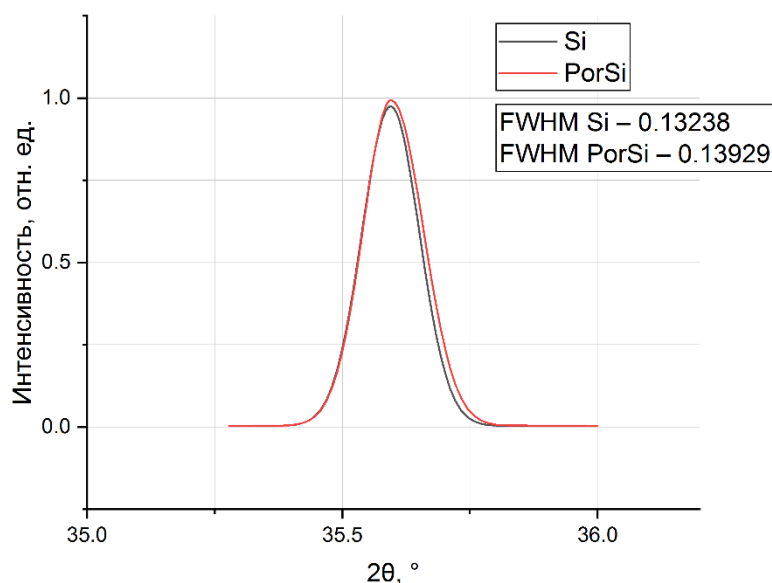
Рис. 1. Профили дифракционных максимумов (111) от исходного монокристаллического кремния и от слоя пористого кремния
