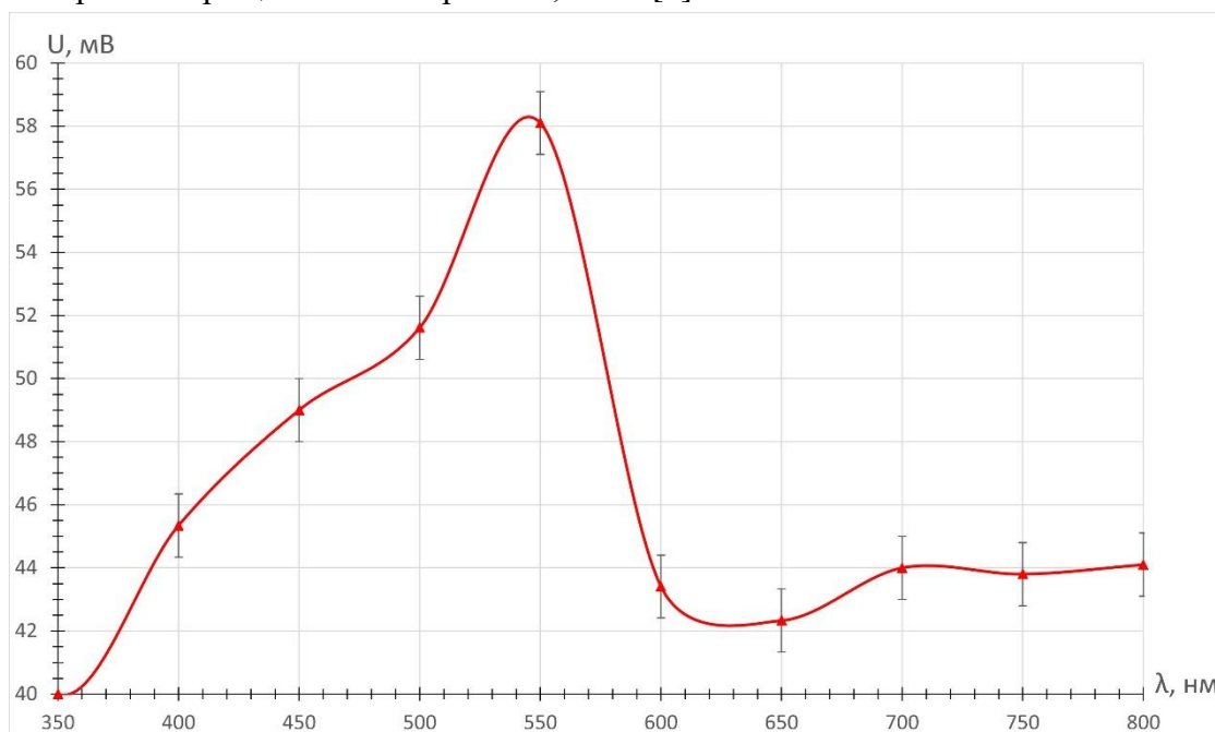
Рис. 1. Спектральная зависимость фотоздс образца с карбидизацией пористого слоя
