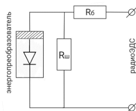
Рис. 1. Эквивалентная схема
