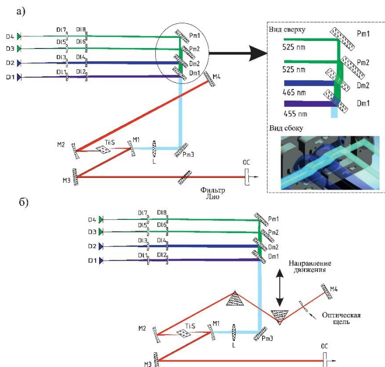
Рис. 1. а) Оптическая схема непрерывного лазера. Блок накачки состоит из четырёх лазерных диодов D1 — D4 , цилиндрических линз Dl1 — Dl8 зеркал накачки Pm1 — Pm3 , дихроичных зеркал Dm1 — Dm2 и сферической линзы. Резонатор лазера включает в себя высоко-отражающие зеркала M\# , фильтр Лию и выходное зеркало OC . (б) Оптическая схема фемтосекундного лазера
