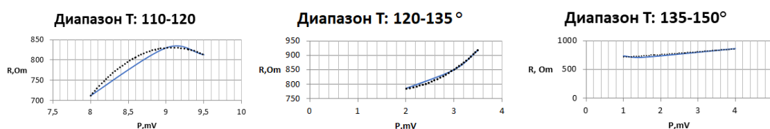
Рисунок 2 – графики зависимости сопротивления от давления при температурах 110-120°C, 120-135°C, 135-150°C.
