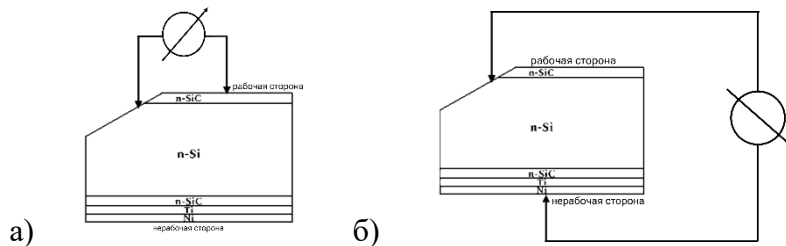
Рис. 2. Схема методики экспериментальных исследований потерь в гетероструктуре SiC/Si с рабочей и нерабочей стороны косого шлифа а) планарное и б) вертикальное исполнение диодной структуры SiC/Si
