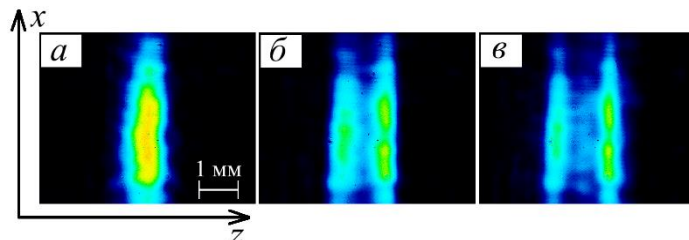
Рис. 1. Изображения профиля пучка, проходящего вдоль оси Y образца \text{LiNbO}_3:\text{Cu} , в моменты времени t = 1 (а), 25 (б), 50 (в)
