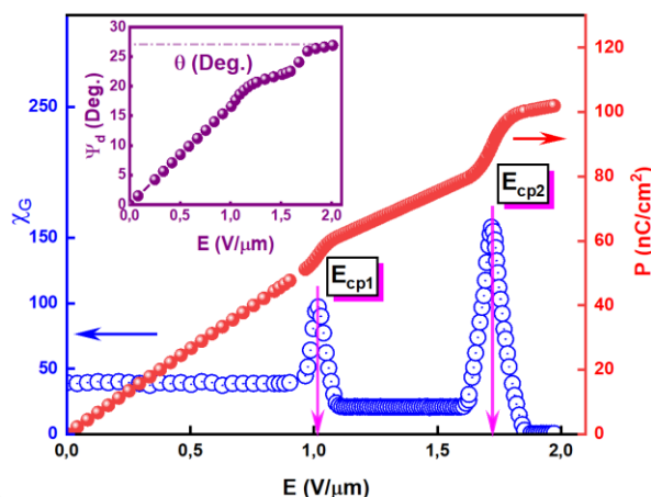
Рисунок 2 – Зависимость поляризации P (красные шарики) и диэлектрической восприимчивости \chi_G (синие кружки) ферриэлектрической смеси нематического ЖК и FODTA-6 от приложенного электрического поля. На вставке зависимость угла отклонения оптической оси \Psi_d ферриэлектрического ЖК (фиолетовые шарики) от электрического поля.
