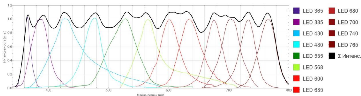
Рис. 1. Относительные спектральные интенсивности светодиодных источников
