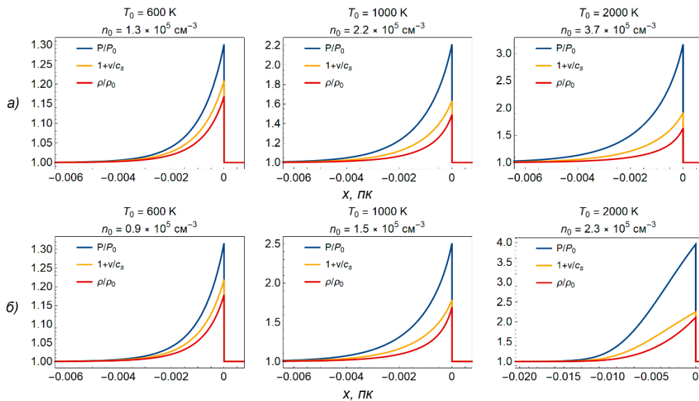
Рис. 1. Профили ударноволновых импульсов при разных стационарных состояниях: а) для функции теплотерь из [2], б) для той же функции с дополнительным учётом нагрева космическими лучами и за счёт фотоионизации С [3]
