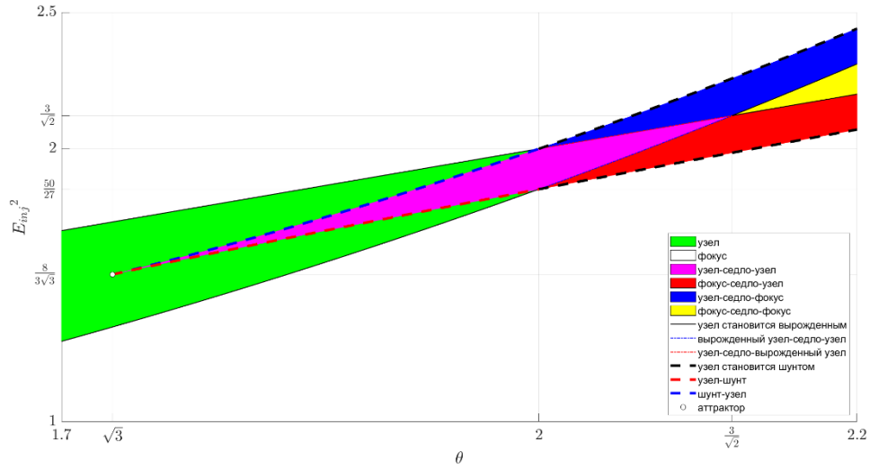
Рис. 1. Бифуркационная диаграмма
