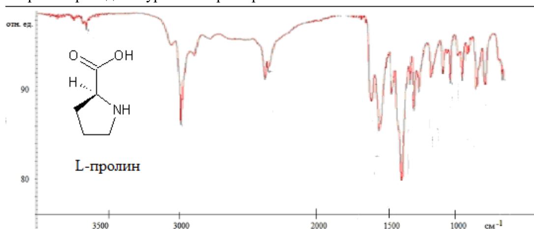
Рис.2. Фурье спектр L_пролина.
