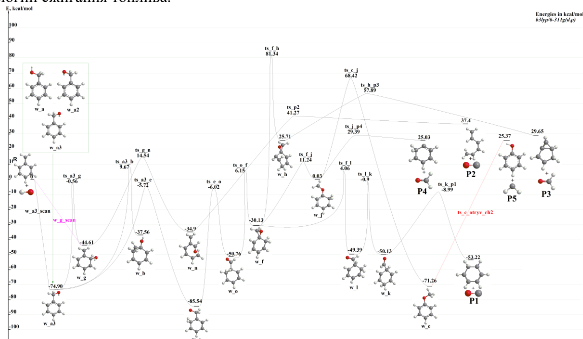
Рис. 1. Поверхность потенциальной энергии реакции C_7H_7 + OH
