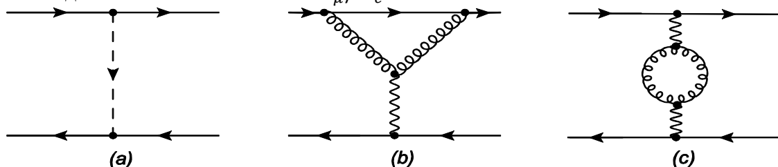
Рис. 1. Амплитуда однобозонного взаимодействия и однофотонного взаимодействия с вершинной и собственно-энергетической поправкой. Пунктирная линия обозначает Z-бозон, волнистая линия обозначает фотон.
