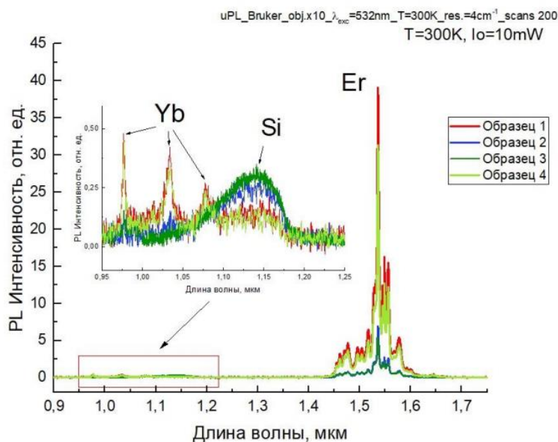
Рис. 1. Спектры микрофотолюминесценции
