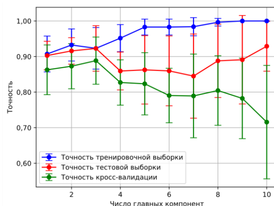
Рис. 1. PLS-DA – Средняя зависимость точности от количества главных компонент с ККО
