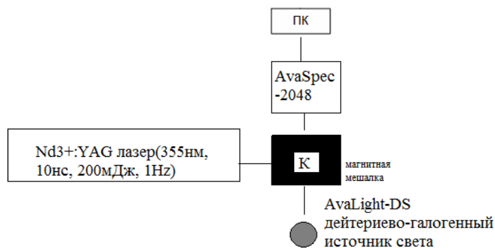
Рис 2. Схема экспериментальной установки. Буквами на рисунке обозначены: К – оптическая кварцевая кювета, ПК – персональный компьютер.
