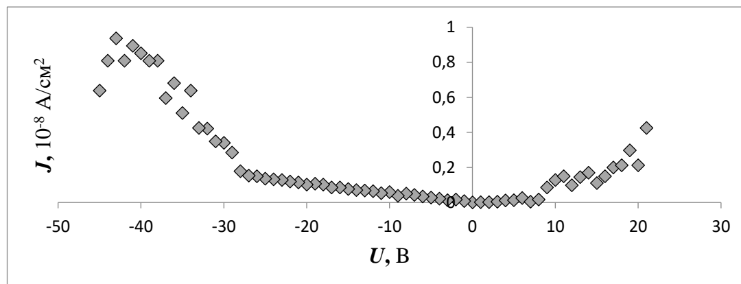
Рис. 1. Зависимость плотности тока от напряжения МДП-структуры Al-SmF 3 -nSi
