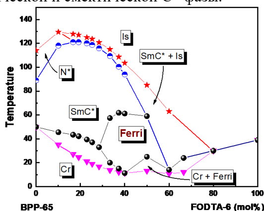
Рисунок 1 – Фазовая диаграмма смеси ахирального смектика С BPP-65 и FODTA-6
