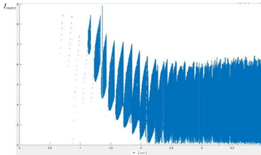
Рис. 1. Бифуркационная диаграмма лазера с обратной связью
