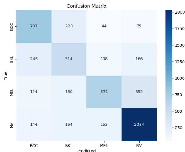
Рисунок 1 – Результаты обучения сети проверенные на тестовом наборе данных
