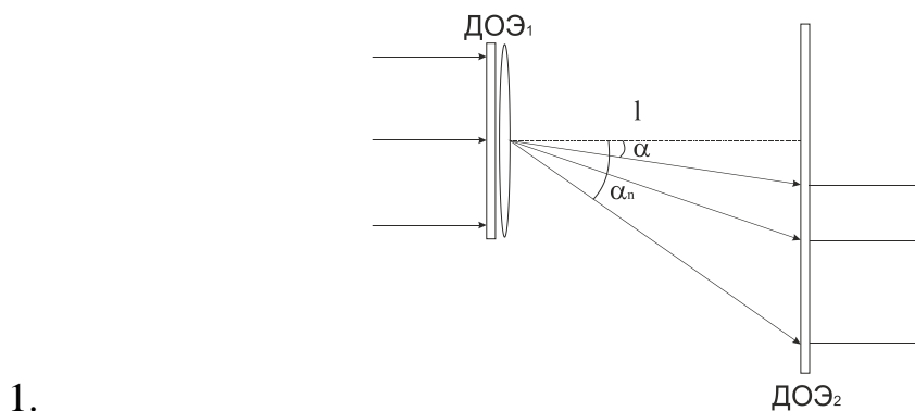
Рис.1. Оптическая схема для многоканальной задержки
