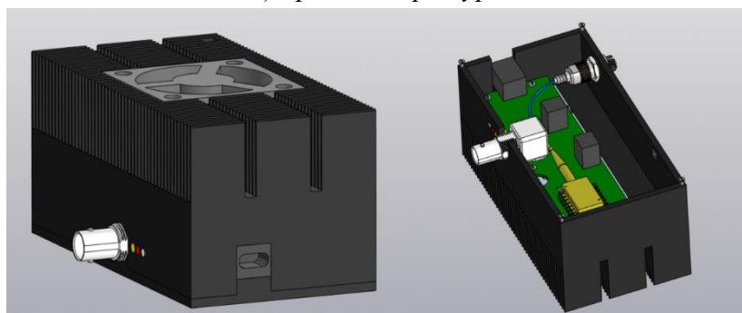
Рис. 2. 3D сборка лазерного модуля
