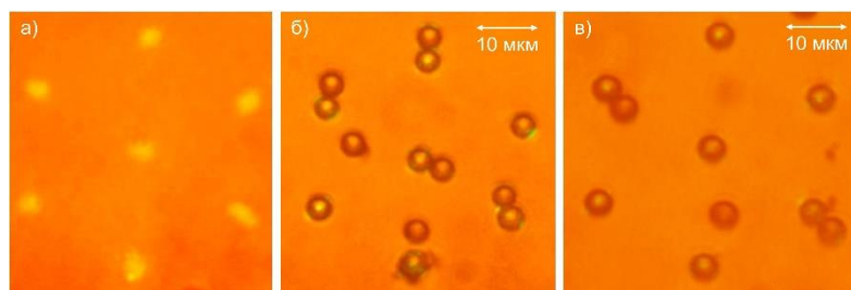
Рис. 1. а) формируемое на эксперименте световое поле, б) захват микросфер в растворе тетрабората натрия, в) захват микросфер в растворе тетрабората натрия с добавлением 40 мМ СДС
