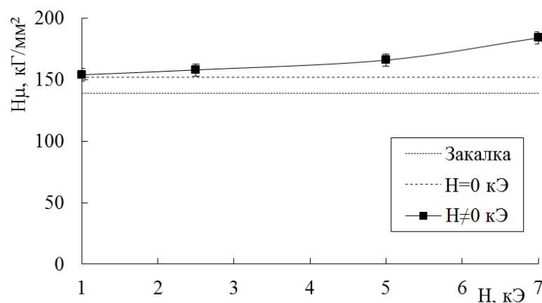
Рис. 1. Полевая зависимость микротвердости состаренного алюминиевого сплава B95пч
