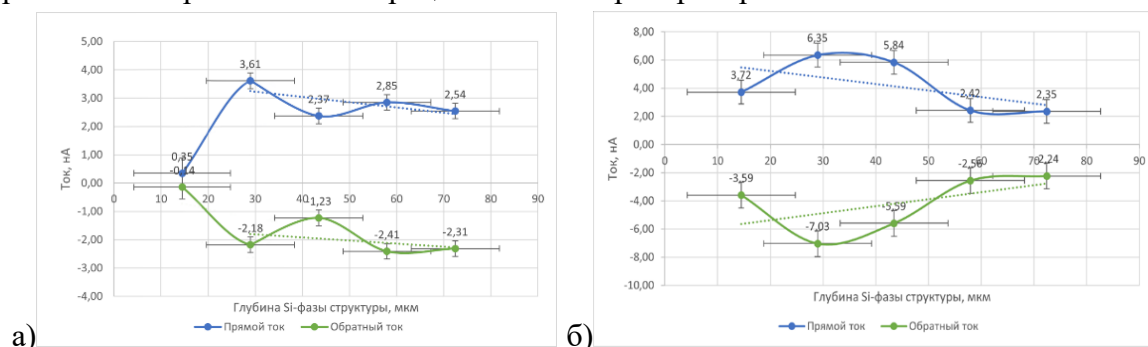
Рис. 3. Графики зависимости тока при сканировании зонда по Si-фазе на косом шлифе в а) планарном и б) вертикальном исполнении диодной структуры SiC/Si
