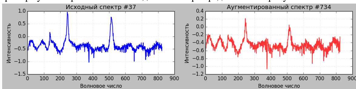
Рис.1 – сравнение исходного и аугментированного спектра
