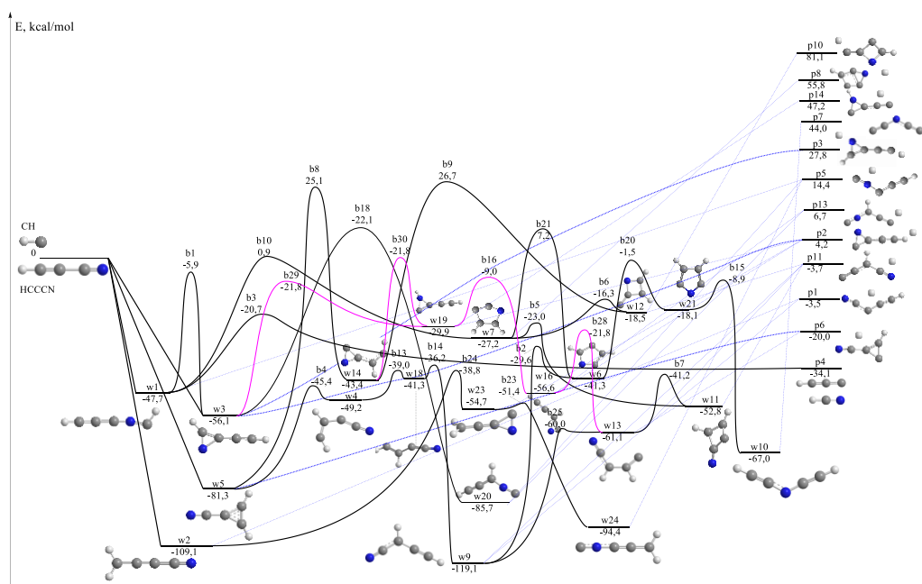
Рис. 1. Поверхности потенциальной энергии цианоацетилена с метиновым радикалом \text{HCCCN} + \text{CH} дополненная новыми реакционными каналами
