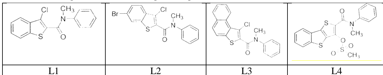
Рис 1. Структурные формулы исследуемых соединений
