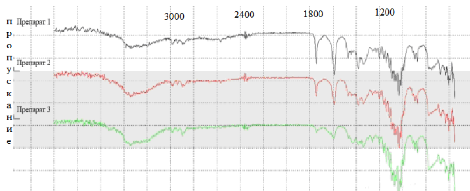
Рис.1. Фурье спектры препаратов каптоприла.
