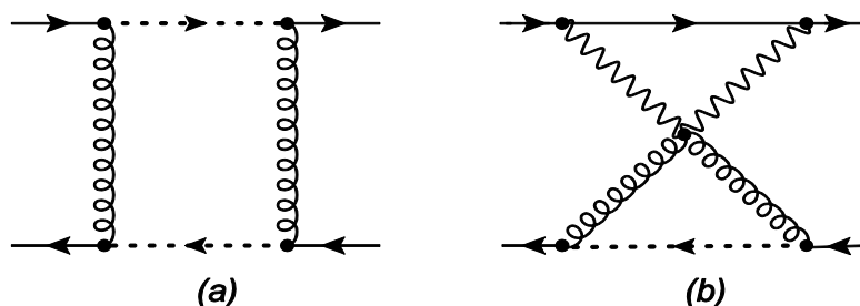
Рис. 3. Амплитуды W -бозонного взаимодействия. Пунктирная линия в промежуточном состоянии обозначает нейтрино.
