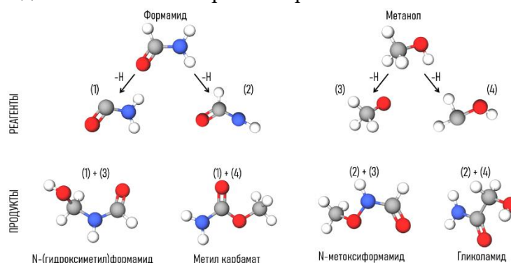
Рис. 1. Реакционная схема синтеза изомеров C_2H_5NO_2 из формамида и метанола
