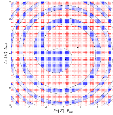
Рис. 2. Бассейны притяжения при |E_{inj}|=2 и \theta=3
