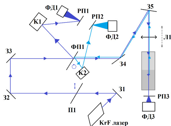
Рис. 1. Экспериментальная схема
